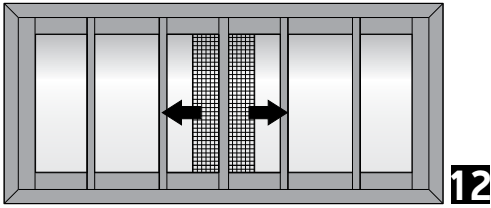
Six sash narrow parallel sliding in 90 assembly window in meeting stile with fly screen Εξάφυλλο Ενάληλη Φιλτρά 90° Κοπή, με σίτα
