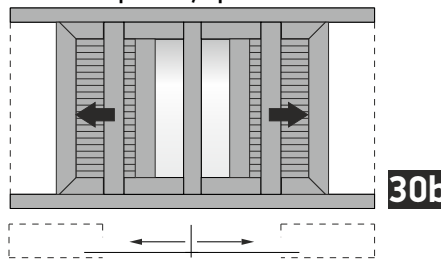
Two-sash pocket sliding window with shutter 90° cut Δίφυλλο χωνευτό με παντζούρι 90° κοπή
