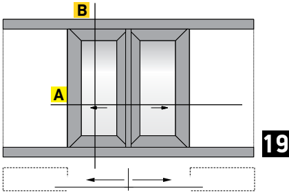
Double sash pocket sliding window in meeting stile Δίφυλλο χωνευτό συρόμενο 45° κοπή
