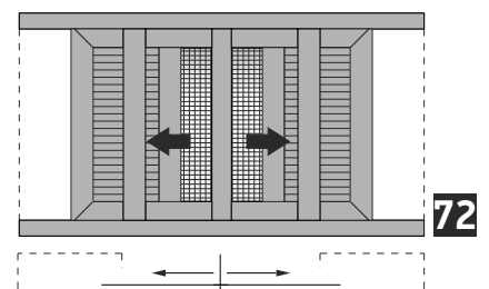
Double narrow sash pocket sliding window in meeting stile, in 90° assembly with glass - fly screens & shutters Δίφυλλο χωνευτό με 90° κοπή, με σήτα και παντζούρι
