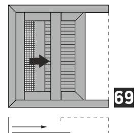
One-sash pocket sliding window 90° cut with glass, fly screen & shutter Μονόφυλλο χωνευτό με 90° κοπή, με σήτα και παντζούρι
