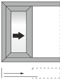
Single sash pocket sliding window Μονόφυλλο χωνευτό συρόμενο 45° κοπή
