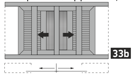
Double narrow sash pocket sliding window in meeting stile, narrow intelocking profile in 90° assembly with glass - fly screens @ shutters Δίφυλλο χωνευτό με 90° κοπή, στενό μπιλί, με σήτα και παντζούρι
