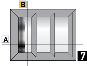
Tribble sash parallel sliding window with fly screen Τρίφυλλο Ενάληθα 45° Κοπή, με σήτα
