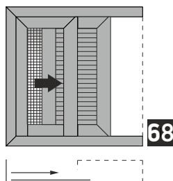
Single sash pocket sliding window in 90° assembly with glass, fly screen & shutter Μονόφυλλο χωνευτό με 90°/45° κοπή στο κάτω/πάνω μέρος του φύλλου, με σήτα και παντζούρι
