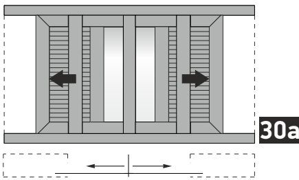
Two-sash pocket sliding window with shutter 90° cut with additional meeting stile Δίφυλλο χωνευτό με παντζούρι 90° κοπή και πρόσθετο μπιλί
