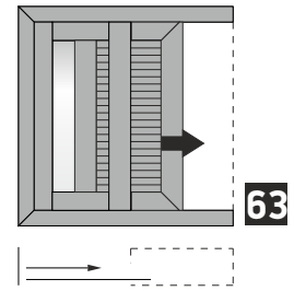
One-sash pocket sliding window 90° cut, with shutter Μονόφυλλο χωνευτό με 90° κοπή, με παντζούρι
