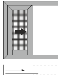
Single sash pocket sliding window in 90° assembly with fly screen Μονόφυλλο χωνευτό με 90°/45° κοπή στο κάτω/πάνω μέρος του φύλλου, με σήτα
