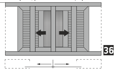
Double sash pocket sliding window in meeting stile, in 90° assembly with glass - fly screens @ shutters Δίφυλλο χωνευτό με 90° κοπή, με σήτα και παντζούρι
