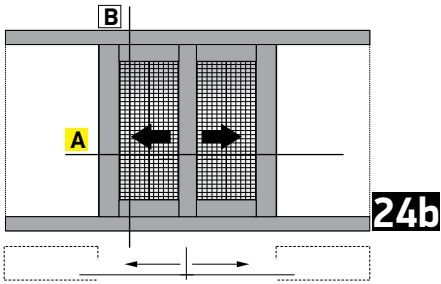
Double sash pocket sliding window 90° cut with narrow meeting stile, with flyscreen Δίφυλλο χωνευτό με 90° κοπή και στενό μπινι, με σήτα
