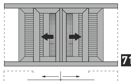
Double sash pocket sliding window in meeting stile, in 90° assembly with glass - fly screens & shutters Δίφυλλο χωνευτό με 90°/45° κοπή στο κάτω/πάνω μέρος του φύλλου, με σήτα και παντζούρι
