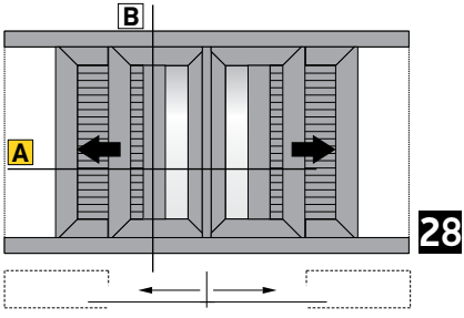
Double sash pocket sliding window in meeting stile with shutters Δίφυλλο χωνευτό συρόμενο 45° κοπή, με παντζούρι
