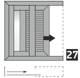
Single sash pocket sliding window 90° cut with shutter Μονόφυλλο χωνευτό με 90° κοπή, με παντζούρι
