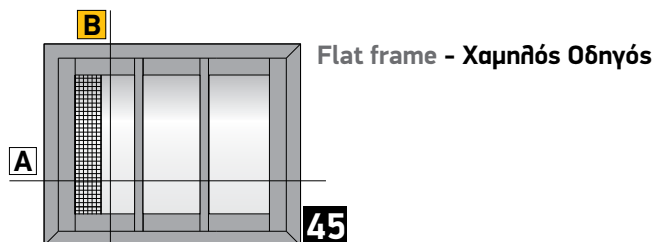
Triple sash narrow parallel sliding window in 90 assembly with fly screen Τρίφυλλο Επάλληλο Συρόμενο με 90° κοπή, με σήτα
