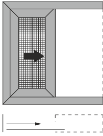
Single sash pocket sliding window with fly screen Μονόφυλλο χωνευτό συρόμενο 45° κοπή, με σήτα
