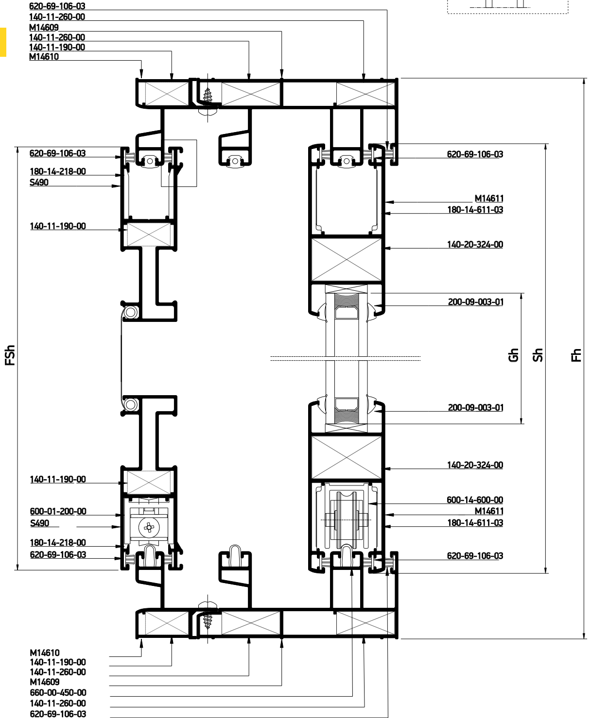
Double sash parallel sliding window with fly screen Δίφυλλο Ενάληθη Συρόμενο 45° κοπή με σίτα
