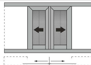
Double sash pocket sliding in 90° assembly window in meeting stile with fly screen Δίφυλλο χωνευτό με 90°/45° κοπή στο κάτω/πάνω μέρος του φύλλου, με σήτα
