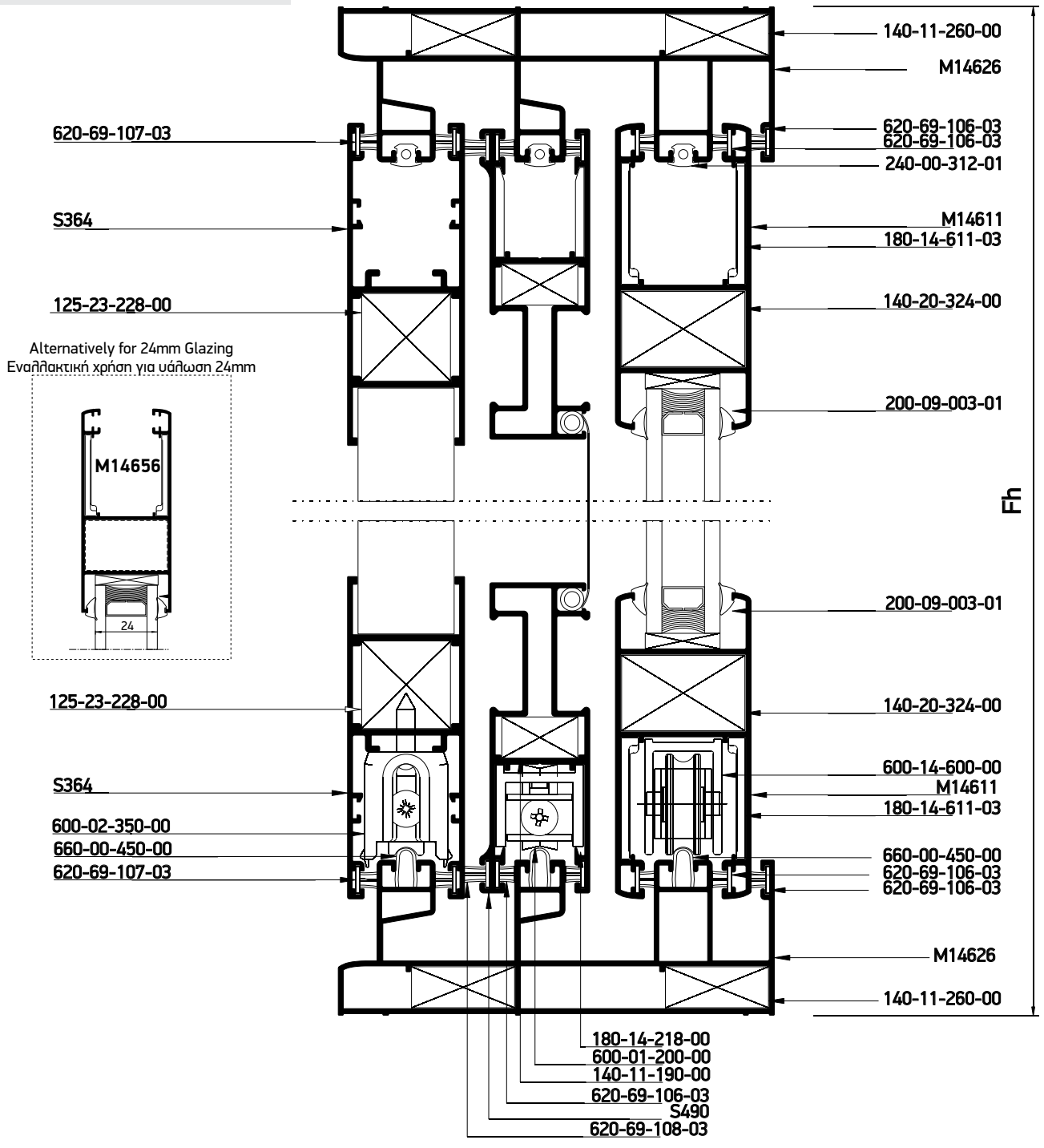
Single sash pocket sliding window with glass - fly screen & shutter Μονόφυλλο χωνευτό συρόμενο 45°κοπή, με σίτα και παντζούρι
