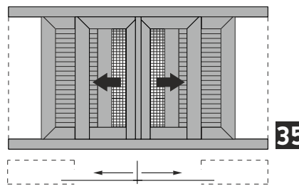
Double sash pocket sliding window in meeting stile, in 90° assembly with glass - fly screens @ shutters Δίφυλλο χωνευτό με 90°/45° κοπή στο κάτω/πάνω μέρος του φύλλου, με σήτα και παντζούρι
