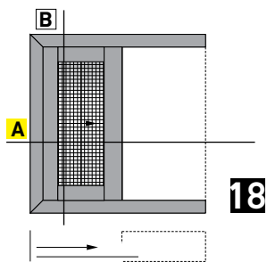
Single sash pocket sliding window in 90° assembly with fly screen Μονόφυλλο χωνευτό με 90° κοπή, με σίτα
