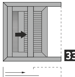
One-sash pocket sliding window 90° cut with flyscreen @ shutter Μονόφυλλο χωνευτό με 90° κοπή, με σήτα και παντζούρι
