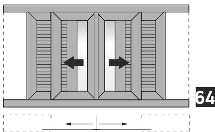
Double sash pocket sliding window 90° in meeting stile with shutters Δίφυλλο χωνευτό συρόμενο 45° κοπή, με παντζούρι
