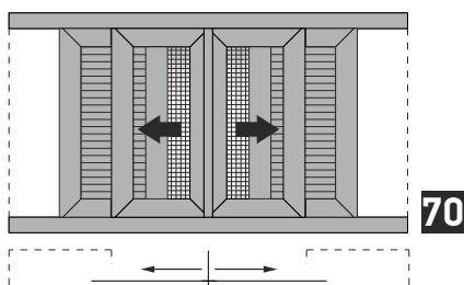
Double sash pocket sliding window in meeting stile, with glass - fly screens & shutters Δίφυλλο χωνευτό συρόμενο 45° κοπή, με σήτα και παντζούρι
