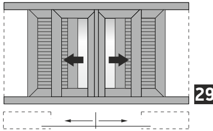
Double sash pocket sliding window in 90° assembly with shutters Δίφυλλο χωνευτό με 90°/45° κοπή στο κάτω/πάνω μέρος του φύλλου, με παντζούρι
