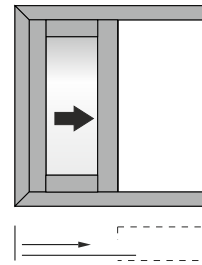
Single narrow sash pocket sliding window in 90°/45° assembly Μονόφυλλο χωνευτό με 90° κοπή
