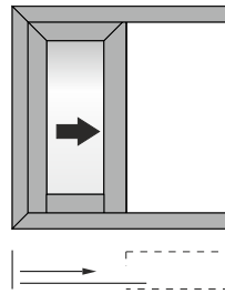
Single sash pocket sliding window in 90°/45° assembly Μονόφυλλο χωνευτό με 90°/45° κοπή στο κάτω/πάνω μέρος του φύλλου
