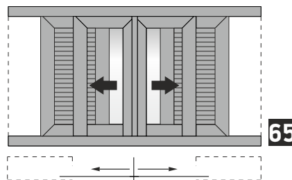
Double sash pocket sliding window in 90° assembly in meeting stile with shutters Δίφυλλο χωνευτό με 90°/45° κοπή στο κάτω/πάνω μέρος του φύλλου, με παντζούρι
