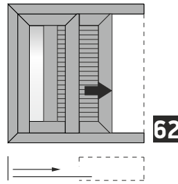
Single sash pocket sliding window in 90° assembly with shutter Μονόφυλλο χωνευτό με 90°/45° κοπή στο κάτω/πάνω μέρος του φύλλου, με παντζούρι
