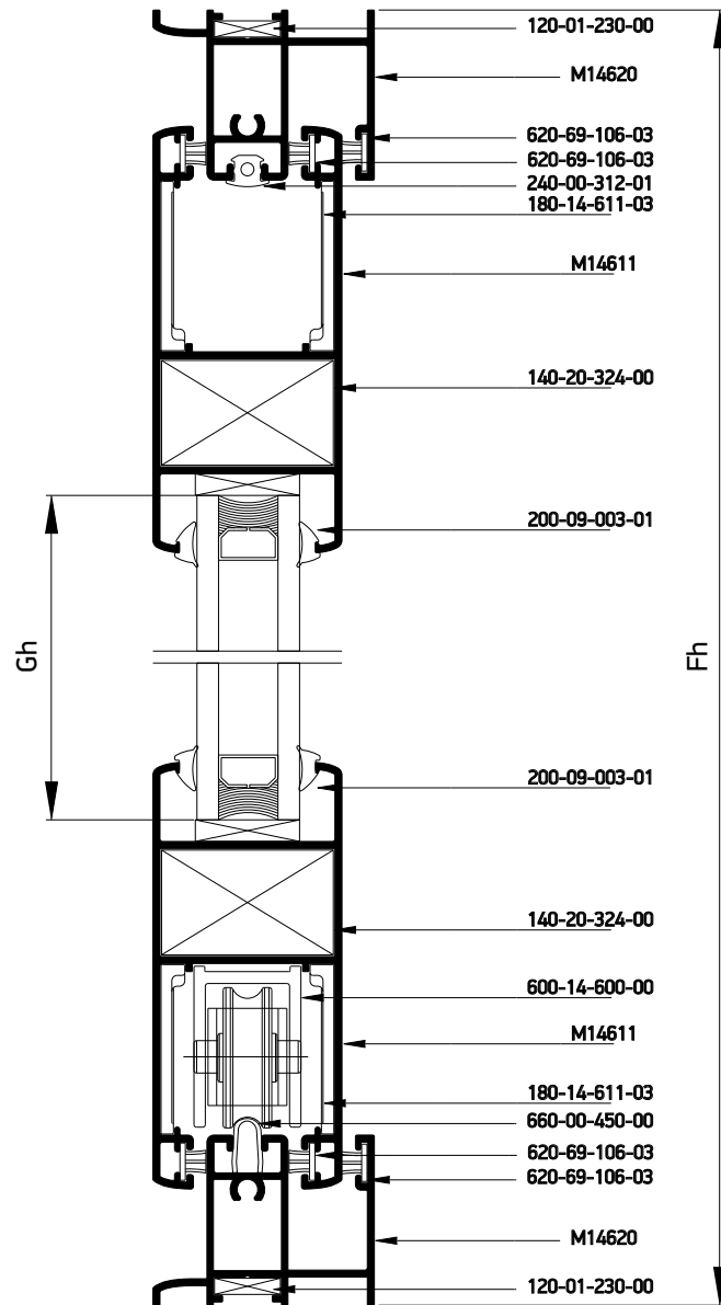
Single sash pocket sliding window Μονόφυλλο χωνευτό συρόμενο 45° κοπή
