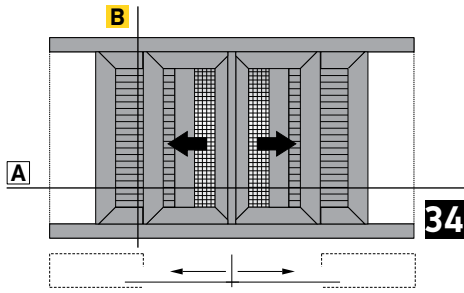
Double sash pocket sliding window in meeting stile, with glass - fly screens & shutters Δίφυλλο χωνευτό συρόμενο 45° κοπή, με σήτα και παντζούρι
