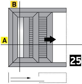
Single sash pocket sliding window with shutter Μονόφυλλο χωνευτό συρόμενο 45° κοπή με παντζούρι
