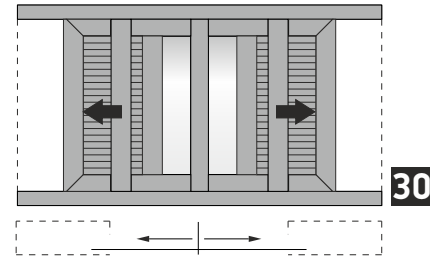
Double sash pocket sliding window with shutter 90° cut with additional meeting stile Δίφυλλο χωνευτό με 90° κοπή και πρόσθετο μπιλί
