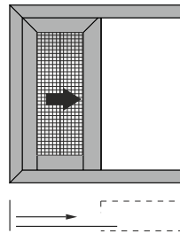
Single sash pocket sliding window in 90°/45° assembly with fly screen Μονόφυλλο χωνευτό με 90°/45° κοπή στο κάτω/πάνω μέρος του φύλλου, με σήτα
