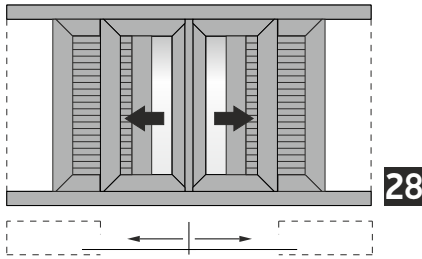
Double sash pocket sliding window in meeting stile with shutters Δίφυλλο χωνευτό συρόμενο 45° κοπή, με παντζούρι
