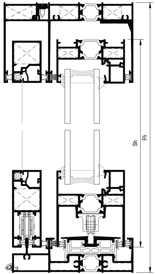
17 Δίφυλλο φιλητό χωνευτό με σήτα Two sash with meeting stile pocket window with flyscreen
