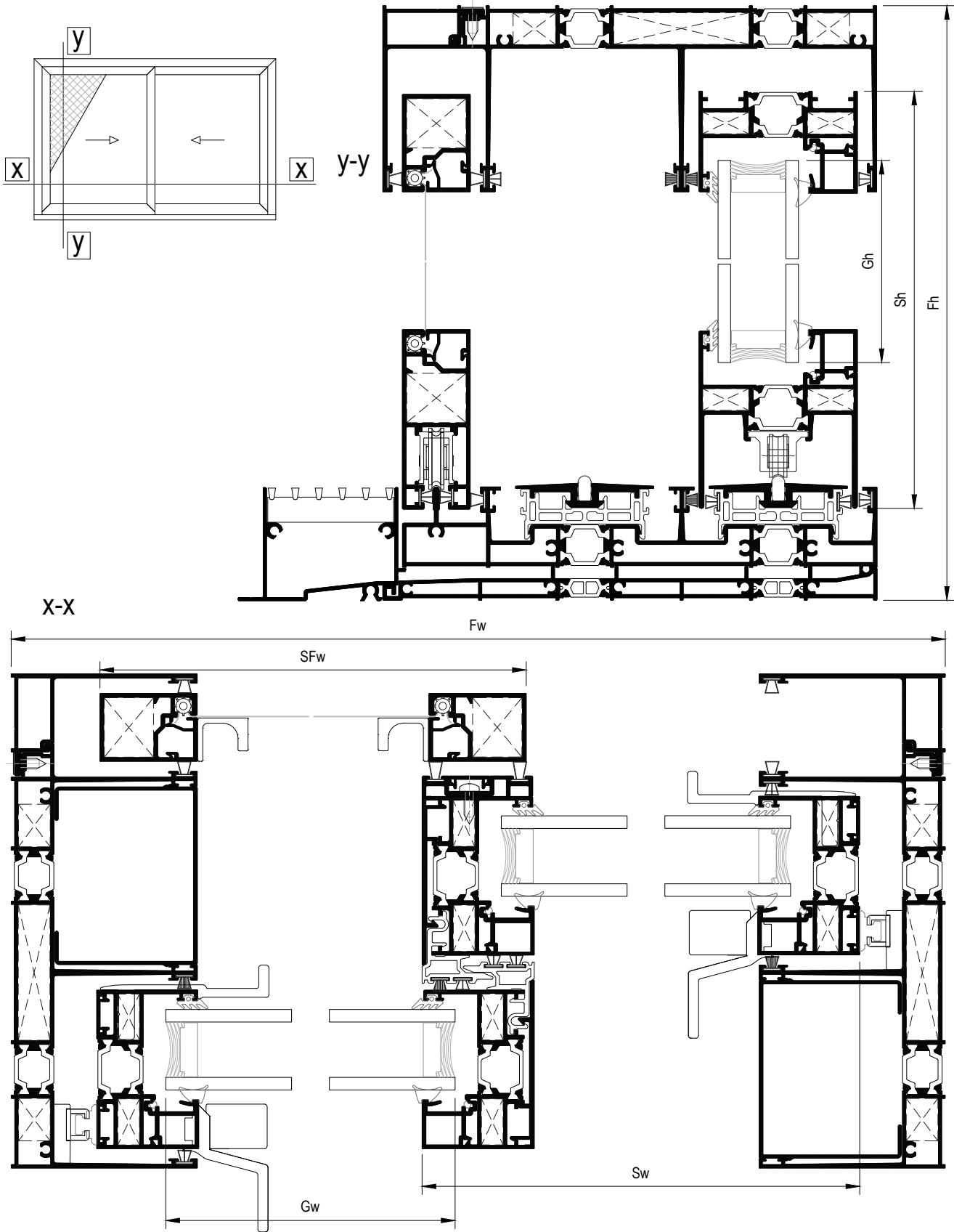
20 Two-sash sliding window with flyscreen and gutter Δίφυλλο επάλληλο συρόμενο με σήτα και υδατολεκάνη
