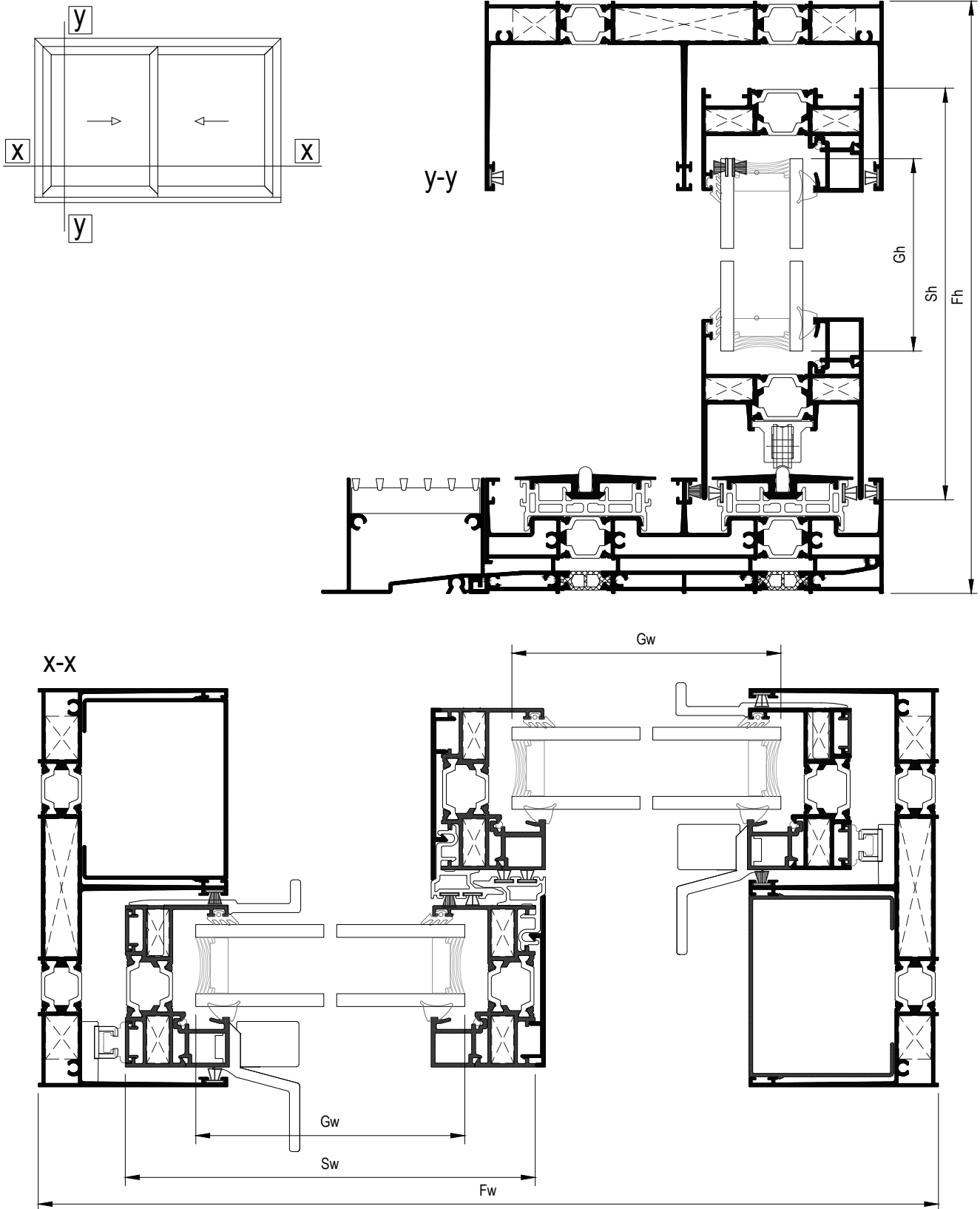
19 Two-sash sliding window with gutter Δίφυλλο επάλληλο συρόμενο με υδατολεκάνη
