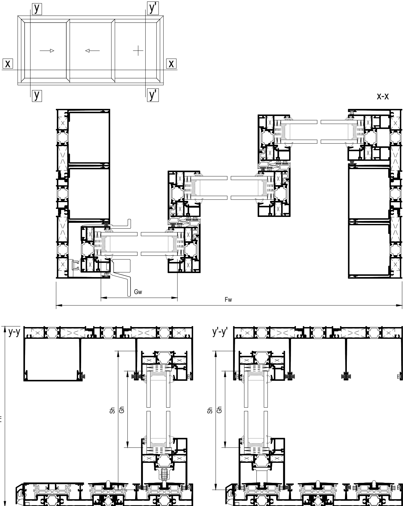
6 Three-sash parallel sliding window with one fixed Τρίφυλλο επάλληλο συρόμενο με σταθερό
