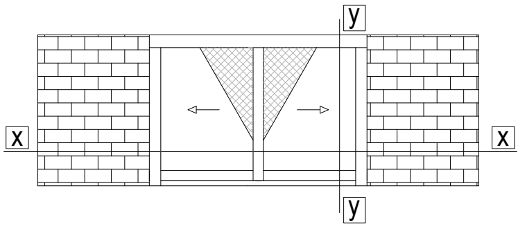
17 Δίφυλλο φιλητό χωνευτό με σήτα Two sash with meeting stile pocket window with flyscreen
